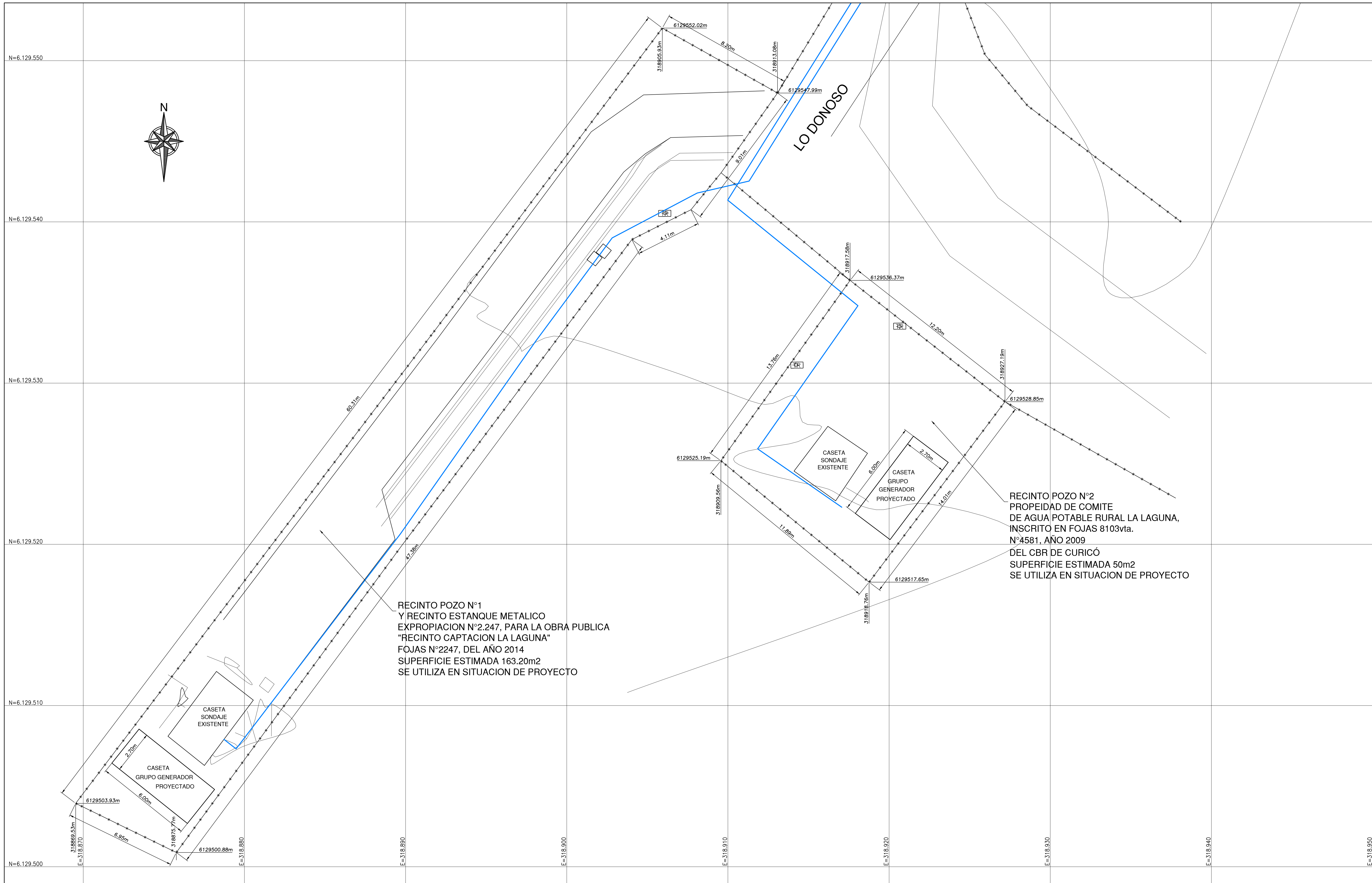
PLANTA RECINTO CAPTACION 1 Y 2 EXISTENTE ESCALA 1 : 100
